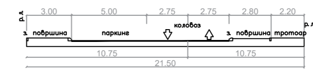
попечни профил А - А
